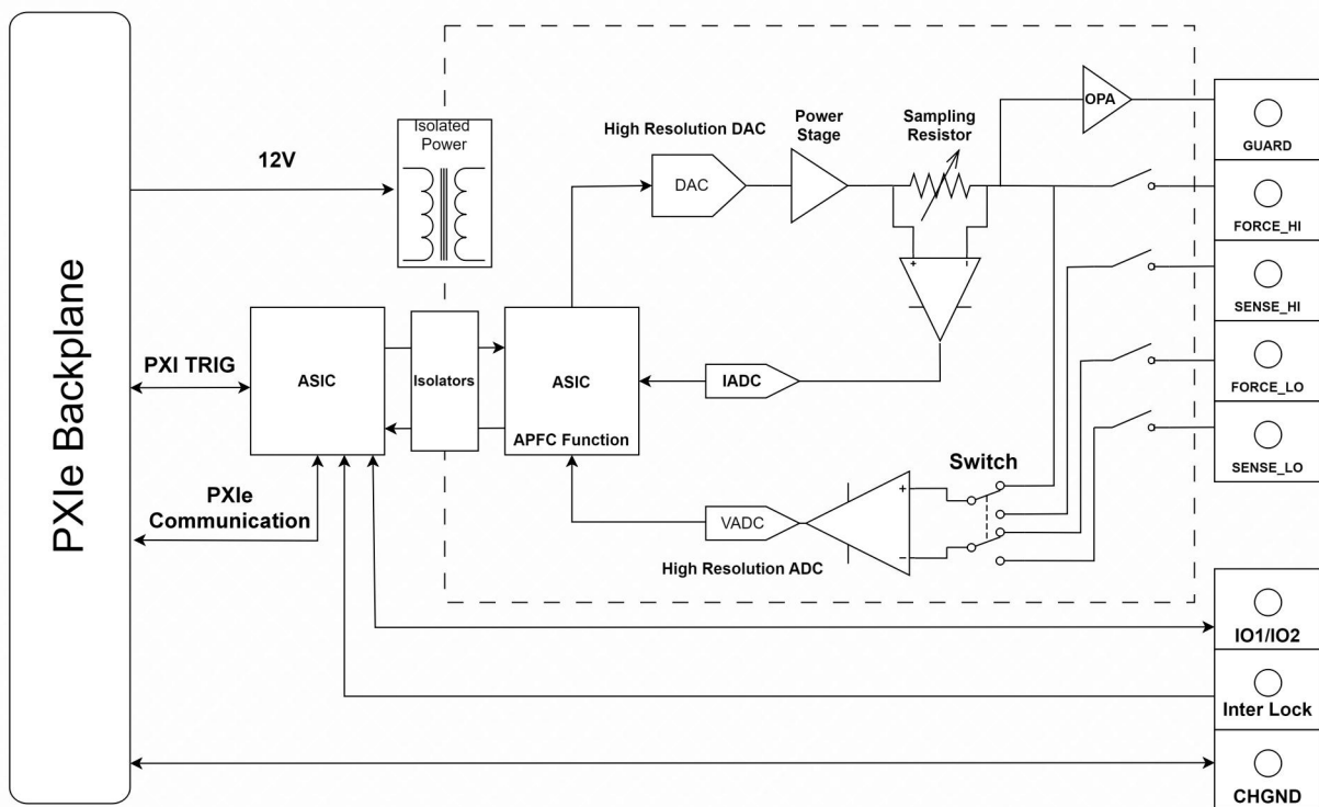
S2013C 架构图
