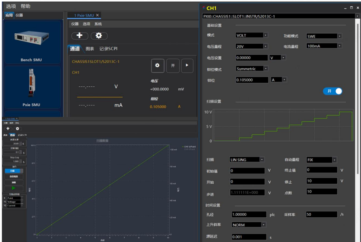
GUI 界面
